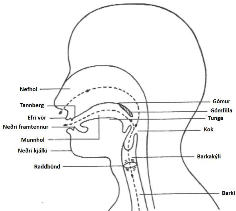
Mynd 11: Talfærin
